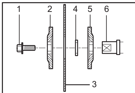
► 1. Boulon hexagonal 2. Bague externe 3. Lame 4. Bague 5. Bague interne 6. Axe
