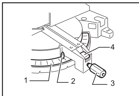
► 1. Échelle de coupe d'onglet 2. Index 3. Poignée 4. Levier de verrouillage
