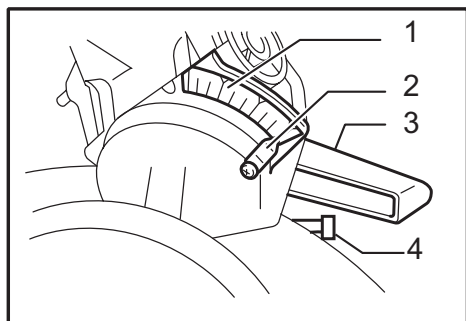
► 1. Échelle de coupe en biseau 2. Index 3. Levier 4. Boulon de réglage de l'angle de coupe en biseau 45°
