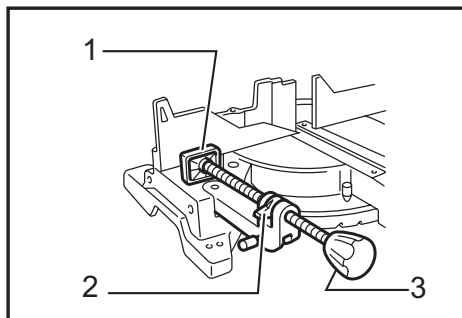
► 1. Vise plate 2. Vise nut 3. Vise knob
